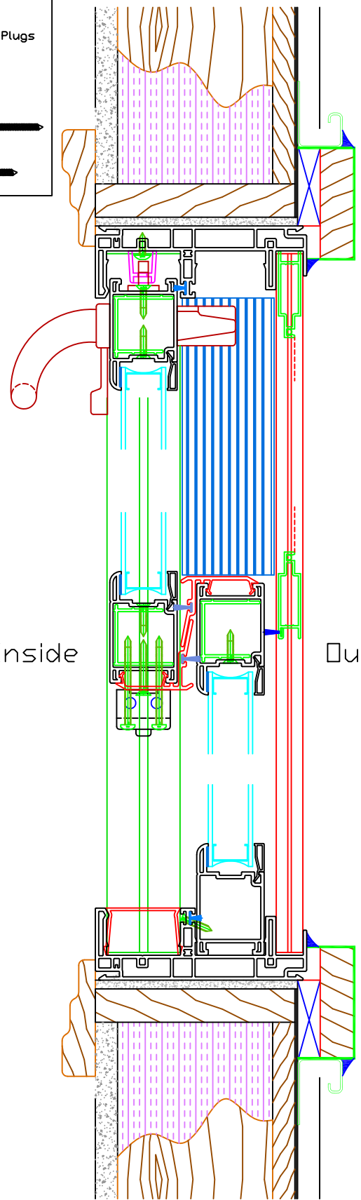
Patio Door Top View
